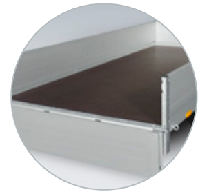
Multiplex-Ladeboden mit Anti-Rutsch-Profil
